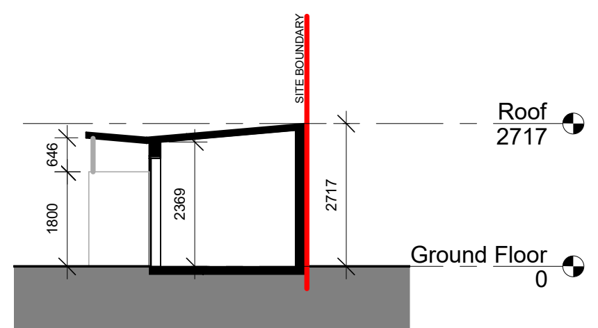
5 Section A-A 1 : 100
