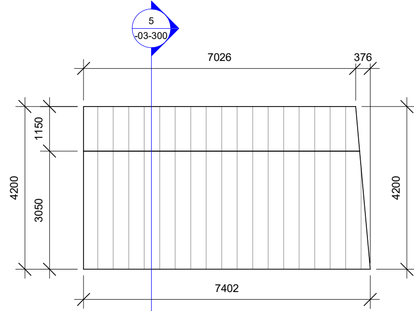
7 Roof 1 : 100
